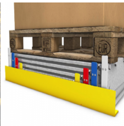
Palettier dynamique
